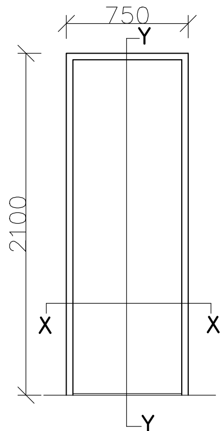
DOOR TYPE D2
